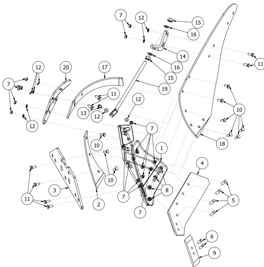
Rysunek R9 PL02924-P18 Kopyto lewe kompletne, odkładnica pełna 18"
