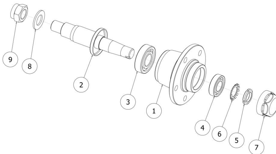
Rysunek R17 PO.EM.00002 Kompletna piasta PO
