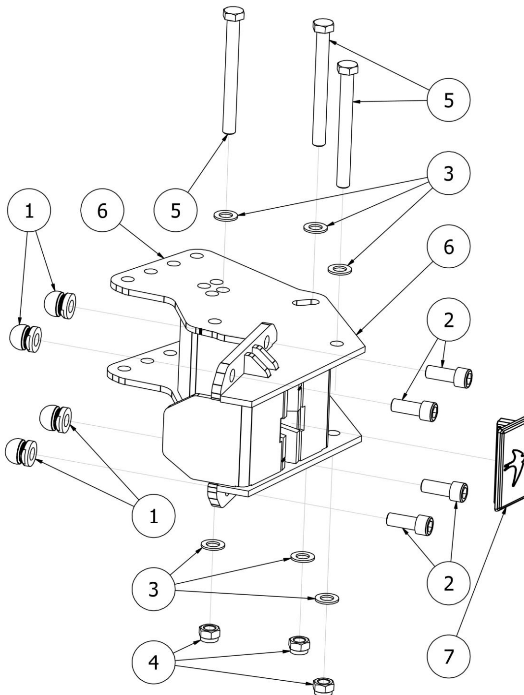
Rysunek R13 | PL03026-02 Kieszek kompletna POR/POH z uchwytem mechanizmu koła
