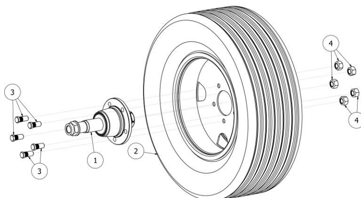
Rysunek R16 PL00456 Koło kompletne
