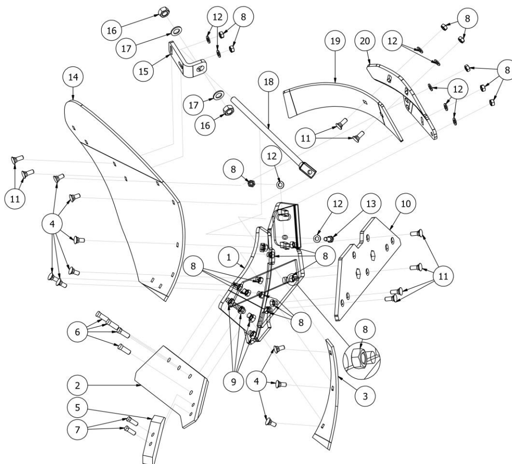
Rysunek R10 | PL02921-P18 Kopyto prawe kompletne, odkładnica pełna 18"
