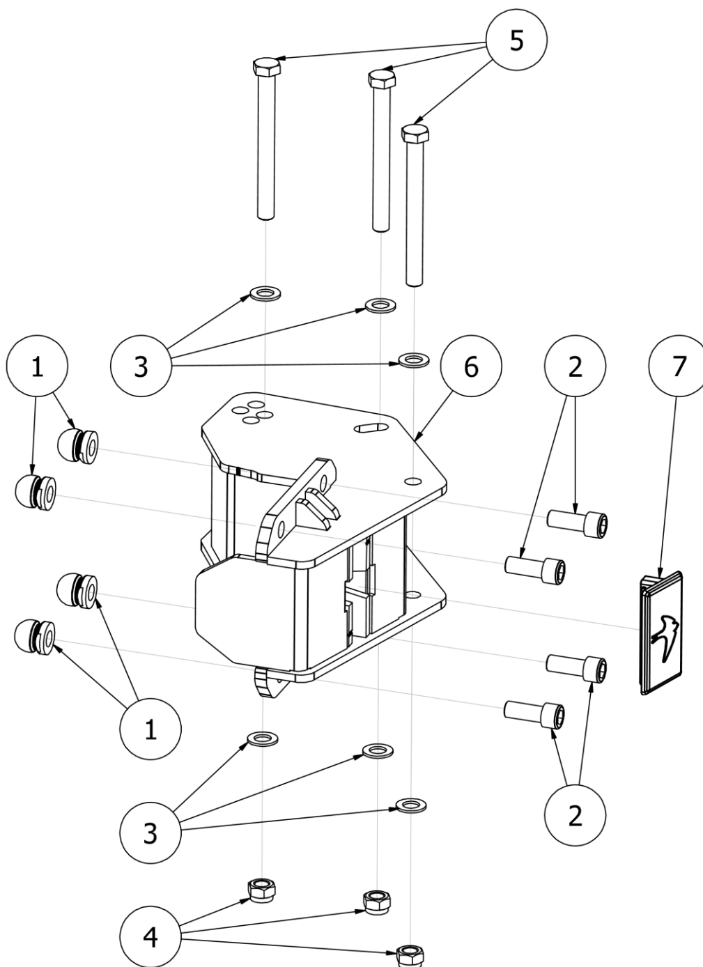
Rysunek R7 PL03026-01 Kieszień kompletna POR/POH
