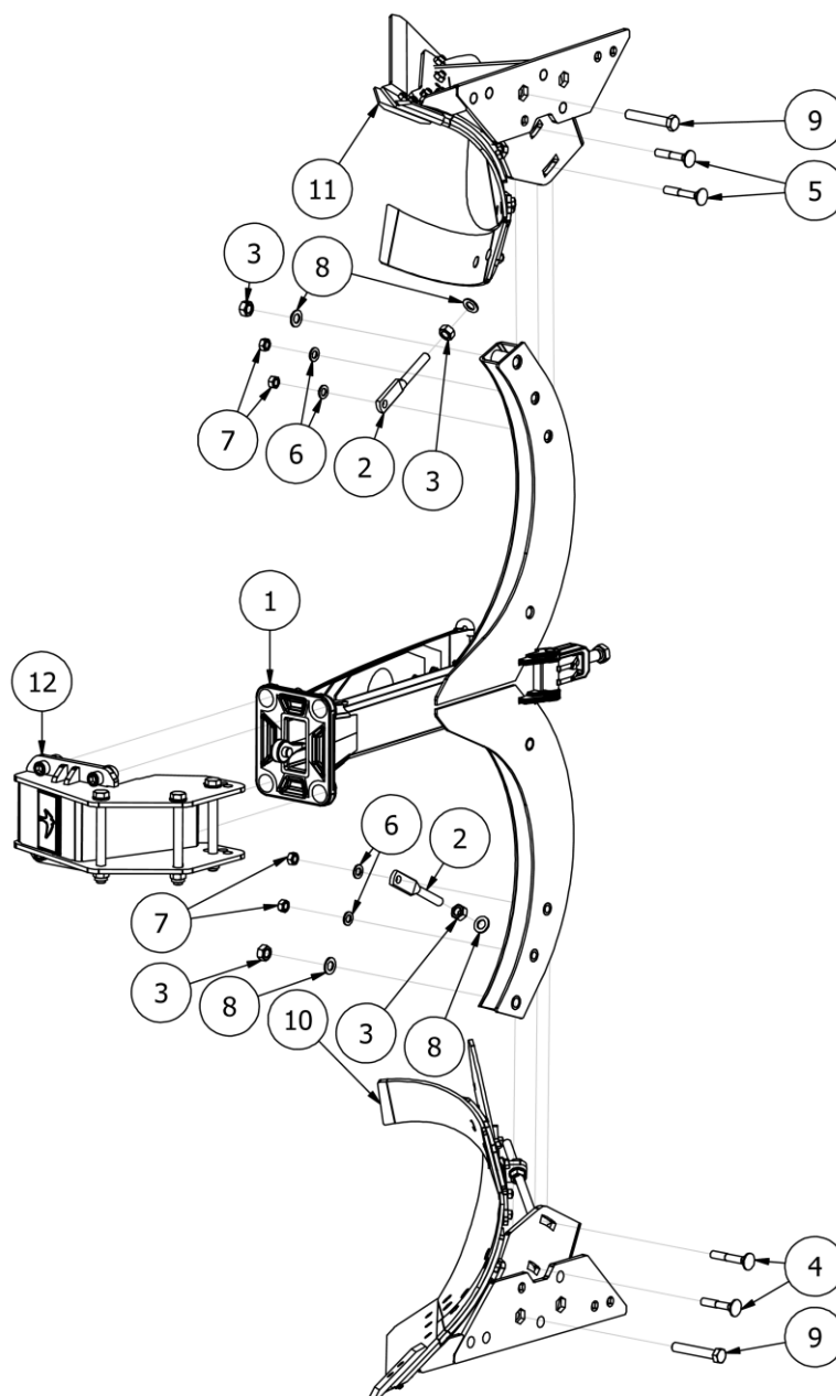
Rysunek R6 PL03023-P18 Korpus kompletny POR, odkładnica pełna
