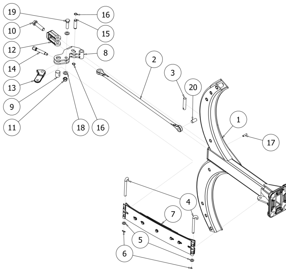
Rysunek R8 PL00374 Ramię kompletne
